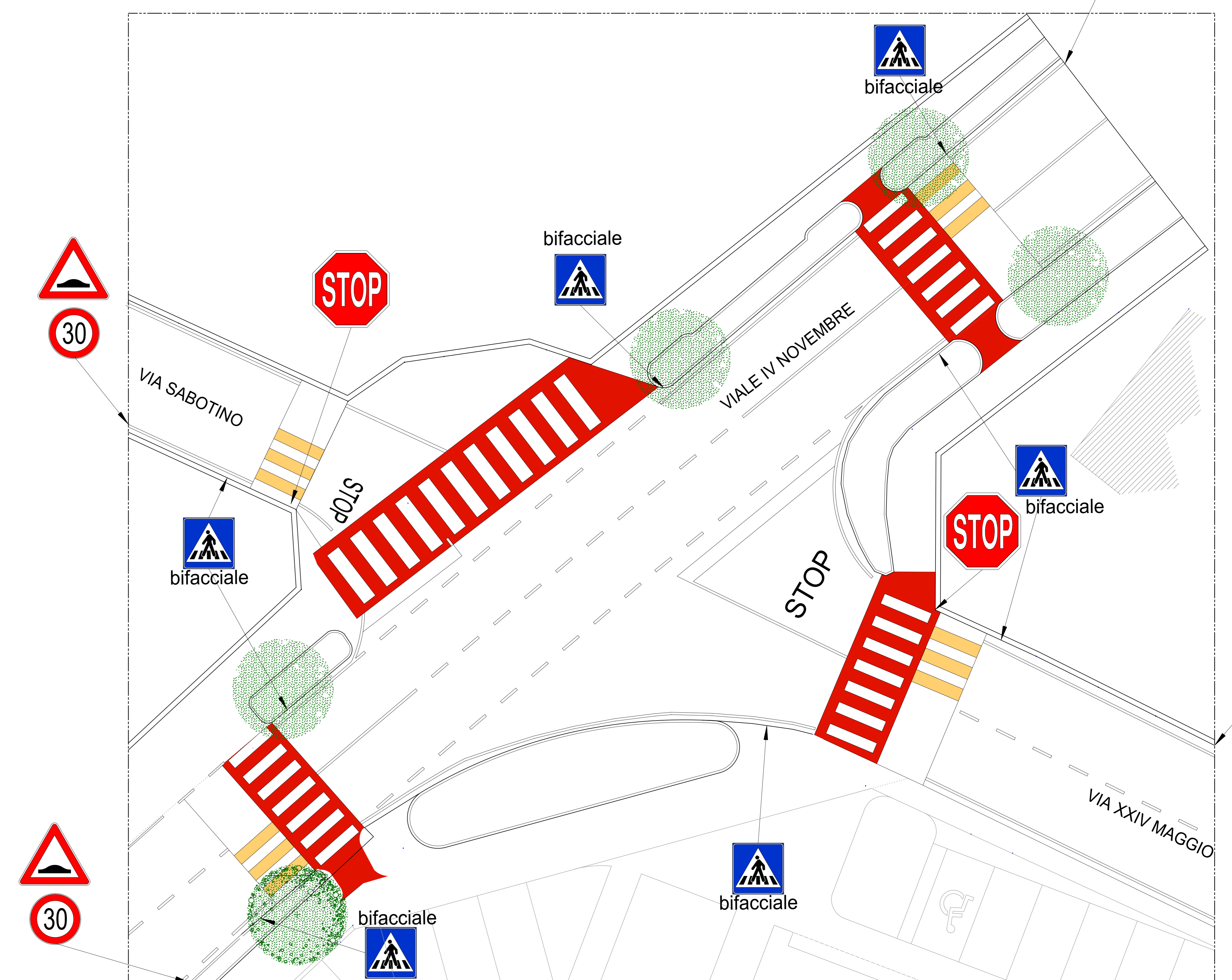
PIANTA DI PROGETTO INTERSEZIONE DA RIQUALIFICARE - SEGNALETICA STRADALE - scala 1:100
